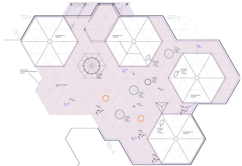
Dach Bestand
