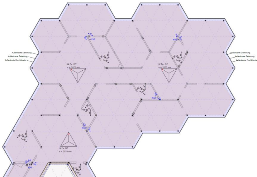
Dach Anbau
